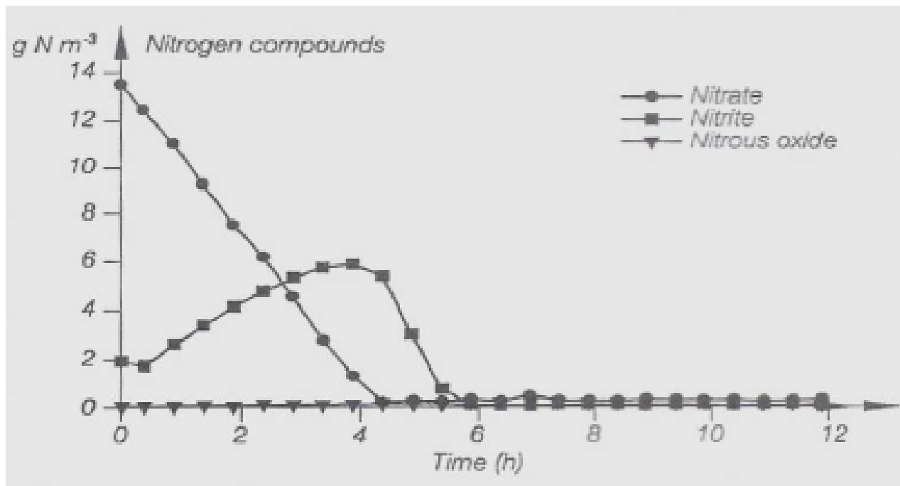
Εικόνα 2.20 Τυπικό προφίλ αναγωγής νιτρικού σε αστικό λύμα δικτύου στους 20^{\circ}\text{C} (Abdul-Talib et al. 2002).
