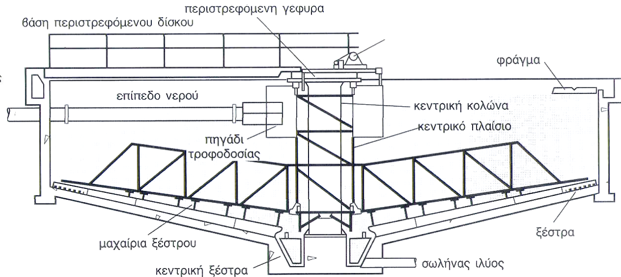
Σχηματικό διάγραμμα παχυντή με βαρύτητα
