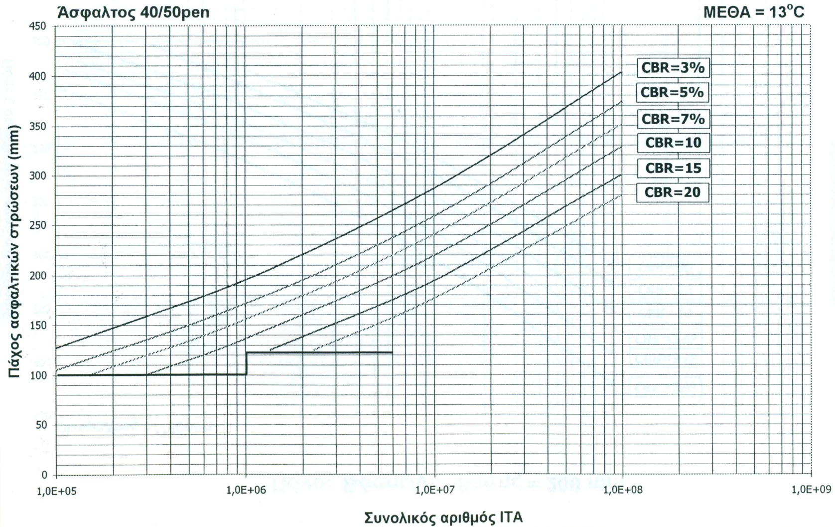
Σχήμα A-8 Νομογράφημα υπολογισμού πάχους ασφαλτικών στρώσεων για πάχος βάσης/υπόβασης 300mm και ΜΕΘΑ 13°C, με άσφαλο 40/50pen
