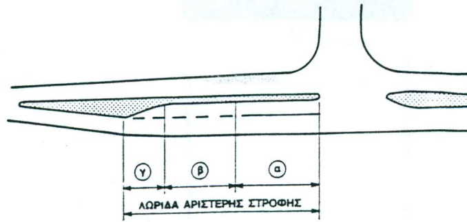
ΣΧΗΜΑ 5.16 Διάταξη λωρίδας άναμονής για άριστερές στροφές.
