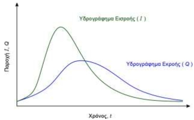
Σχήμα 3.2: Μετασχηματισμός του υδρογραφήματος εισροής σε υδρογράφημα εκροής λόγω της διόδευσης.
