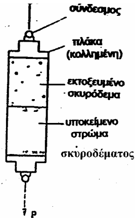
Εικόνα 4-2: Εργαστηριακός Έλεγχος Συνάφειας με Αποκοπή Δείγματος στις περιπτώσεις υποστρώματος με μικρό πάχος
