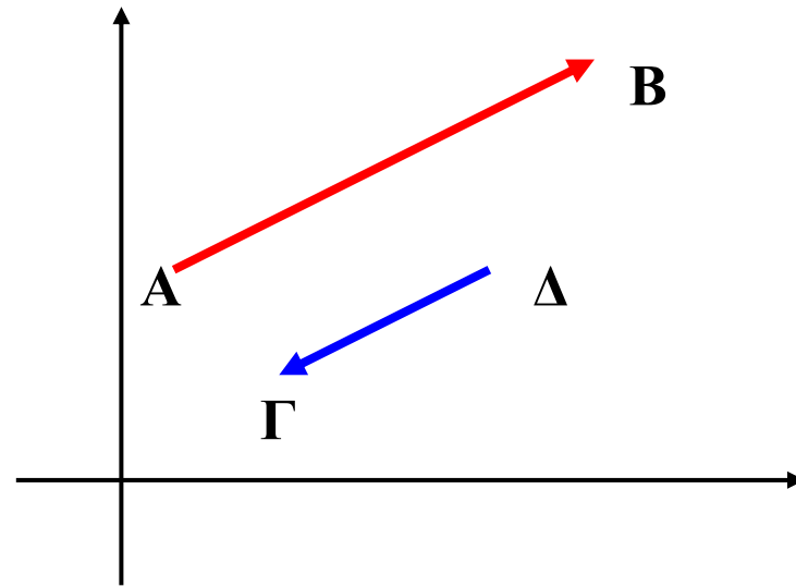
Αντίρροπα διανύσματα
