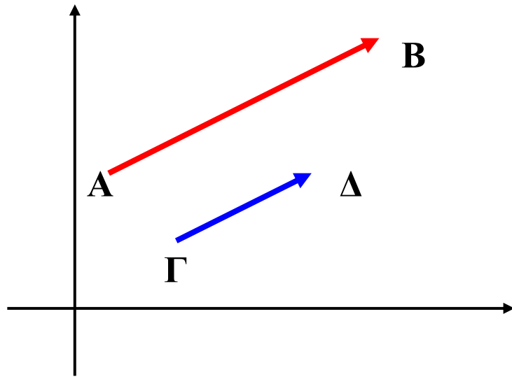
Ομόρροπα διανύσματα
