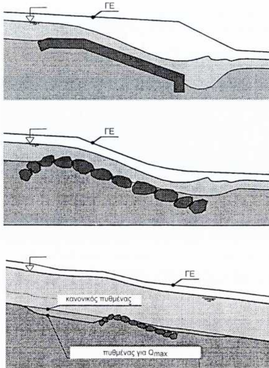
Σχήμα : Συνθήκες ροής σε λεία και σε τραχεία ράμπη
