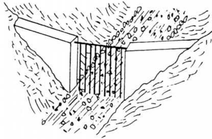
Σχήμα : Φράγμα διαλογής με μεταλλική σχάρα από κατακόρυφες δοκούς
