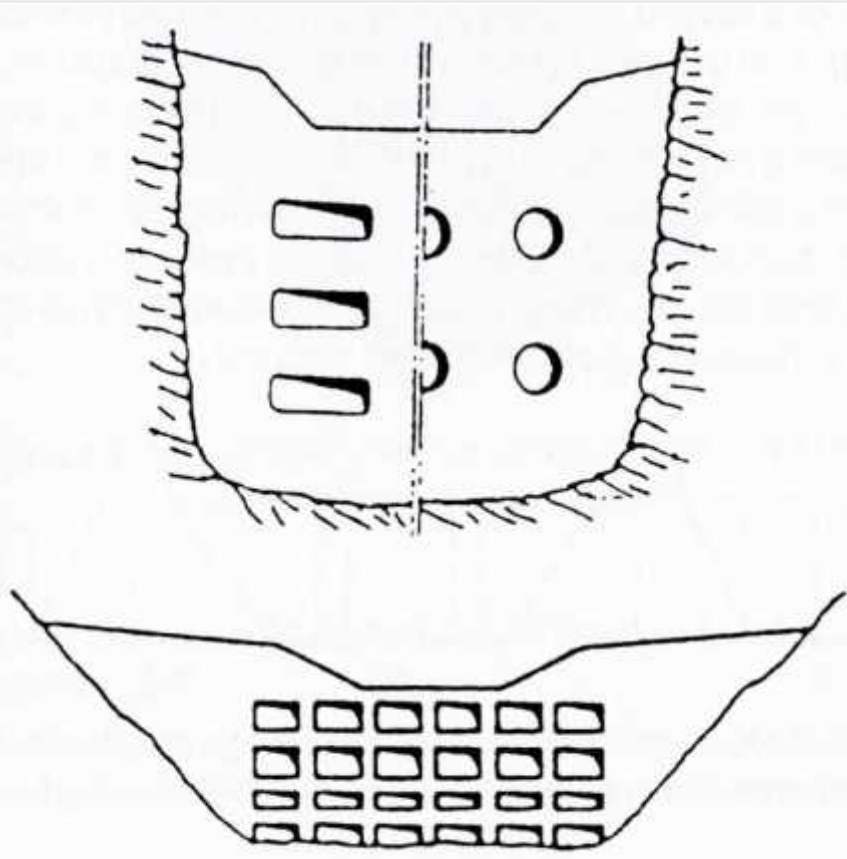
Σχήμα : Φράγμα με μεγαλοχετούς
