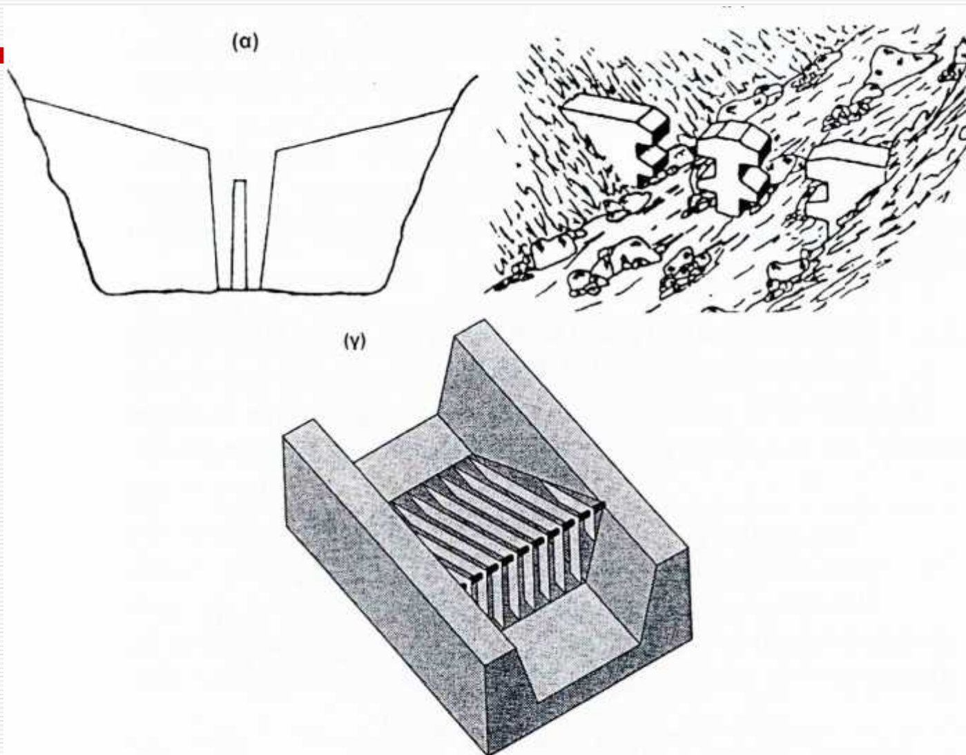
Σχήμα : Φράγματα λαβαθραύσης με προβολικό (α), με ελατόμορφο (β) και με σχαροειδή (γ) λαβαθραυστήρα
