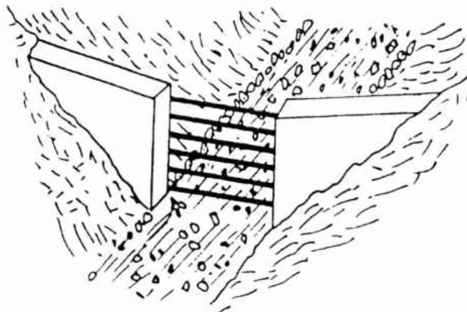
Σχήμα : Φράγμα διαλογής με μεταλλική σχάρα από οριζόντιες δοκούς
