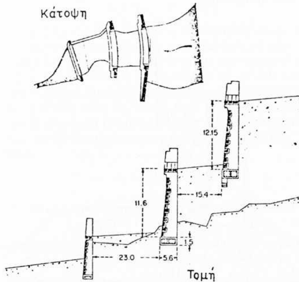
Σχήμα : Διαδοχική σειρά φραγμάτων (σειρά Bretton) για την ανύψωση της κοίτης
