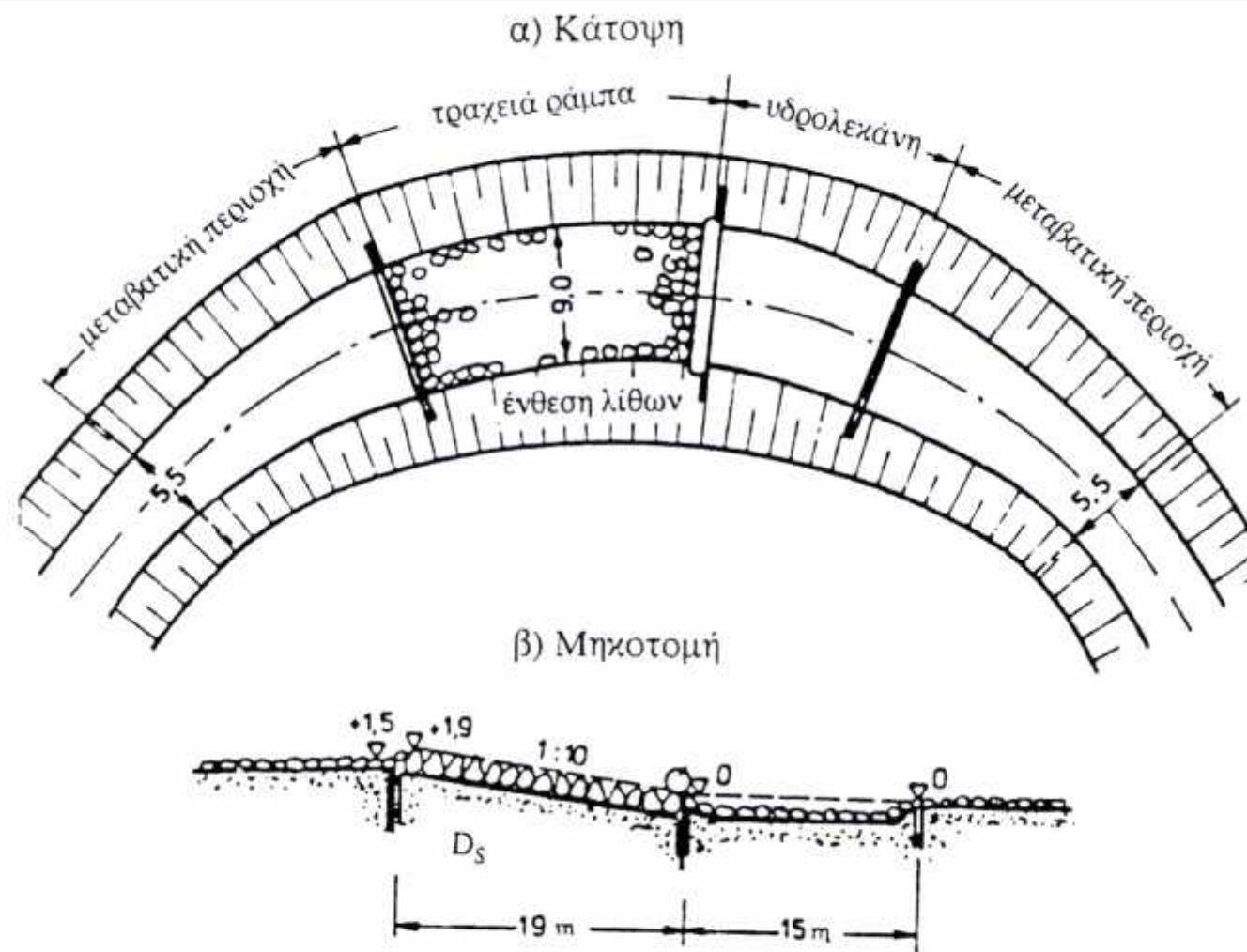
Σχήμα : Υβώδης ουδός με μορφή τραχειάς ράμπας, που κατασκευάστηκε στον ποταμό Kahl
