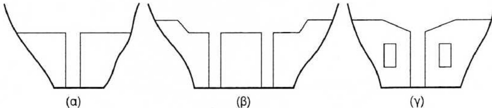
Σχήμα : Φράγμα προσωρινού ελέγχου φερτών υλικών και πλημμυρικών αιχμών με εγκοπή (α), με περισσότερες εγκοπές (β) και με εγκοπή και μεγαλοχετούς (γ)
