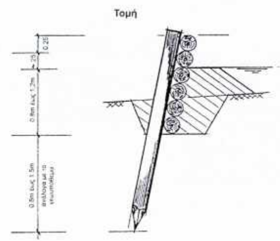
Σχήμα: Ξύλινοι ουδοί σε πρόοψη και τομή
