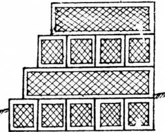
Σχήμα : Τομή ουδού από συρματοπλεκτα κιβώτια.
