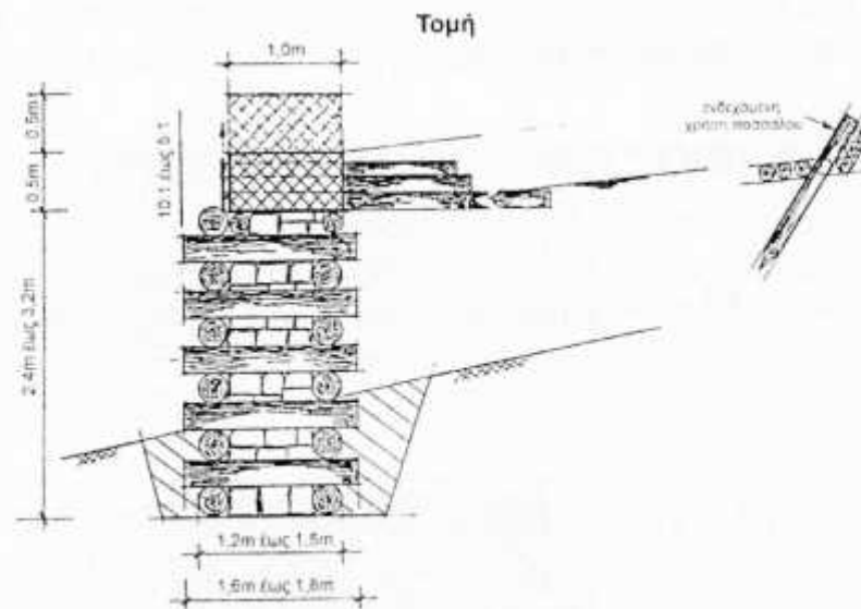
Σχήμα : Μικρό ξυλολιθόφραγμα σε πρόοψη και τομή
