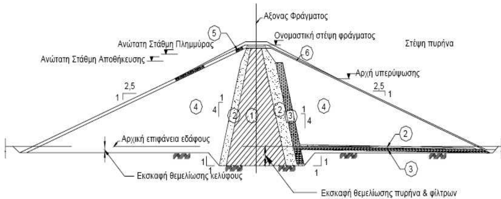
Σχ. 10.1 Τυπική διαζώνηση χωμάτινου φράγματος κε κεντρικό πυρήνα
