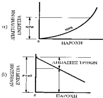
Σχ. 3.31. Παράδοση του υγρού που ρευστό στην περιοχή ικανοποιητικής λειτουργίας μιας αντλίας (α, β, γ: πηλίκι μέτρο, χωρίς αζωδες)
