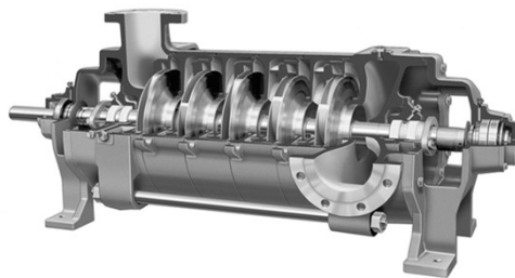
✱ Πολυβάθμια φυγοκεντρική αντλία
