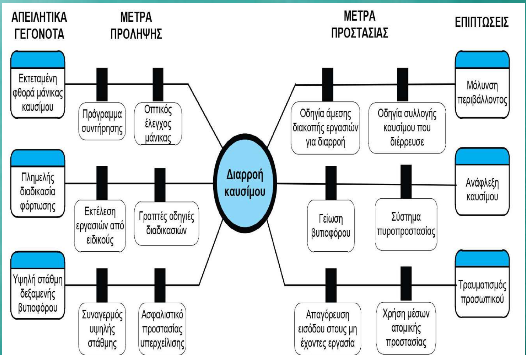
Διάγραμμα Bow-Tie αιτιών και επιπτώσεων για διαρροή καυσίμου
