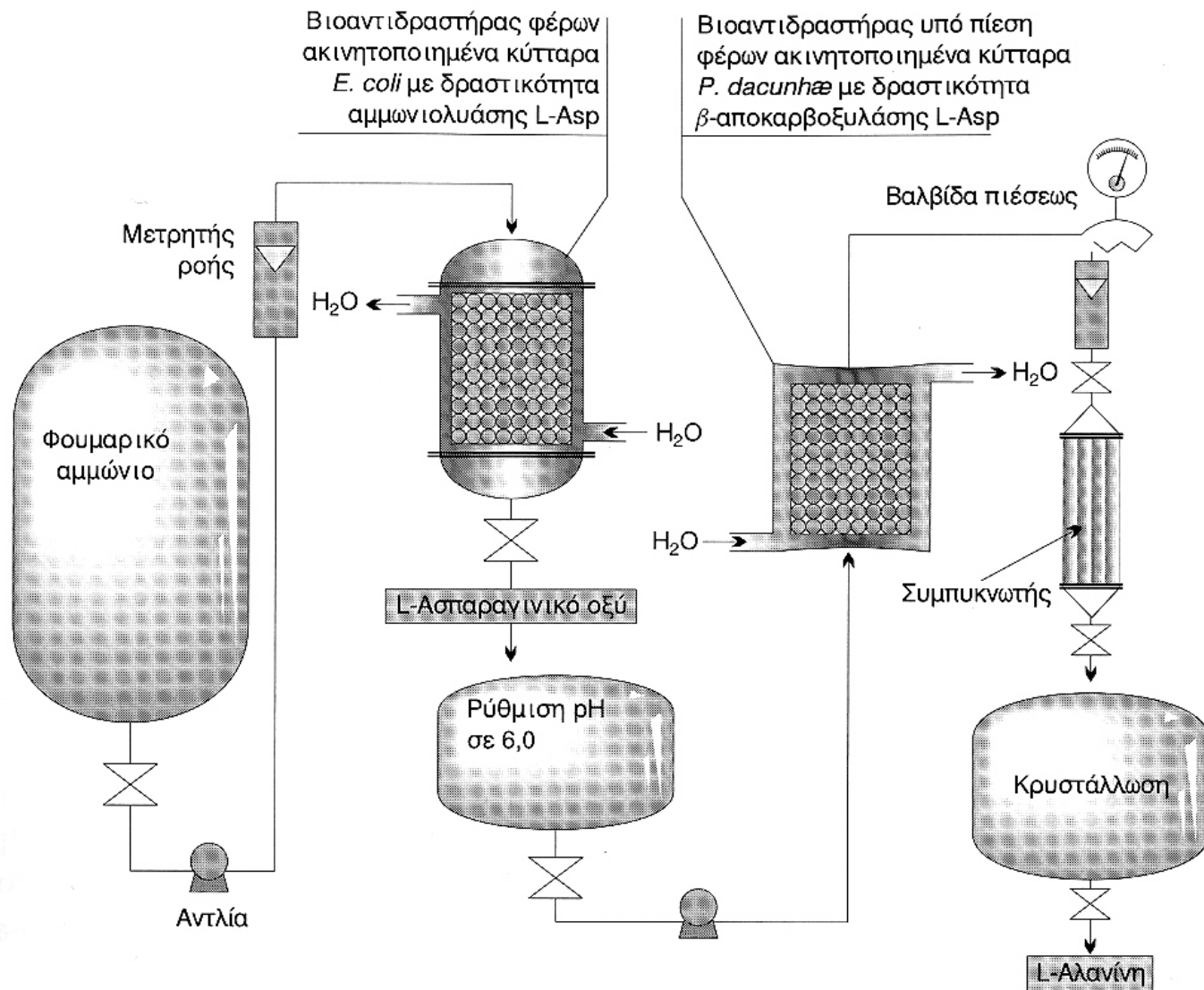
Σχ. 123. Διεργασία παρασκευής L-Asp και L-Ala.
