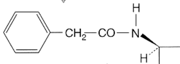
Βενζυλο-πενικιλίνη
