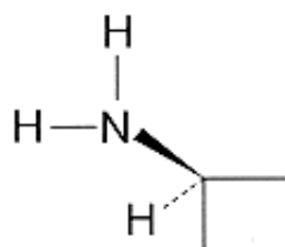
6-Αμινοπενικιλανικό οξύ (6-APA)
