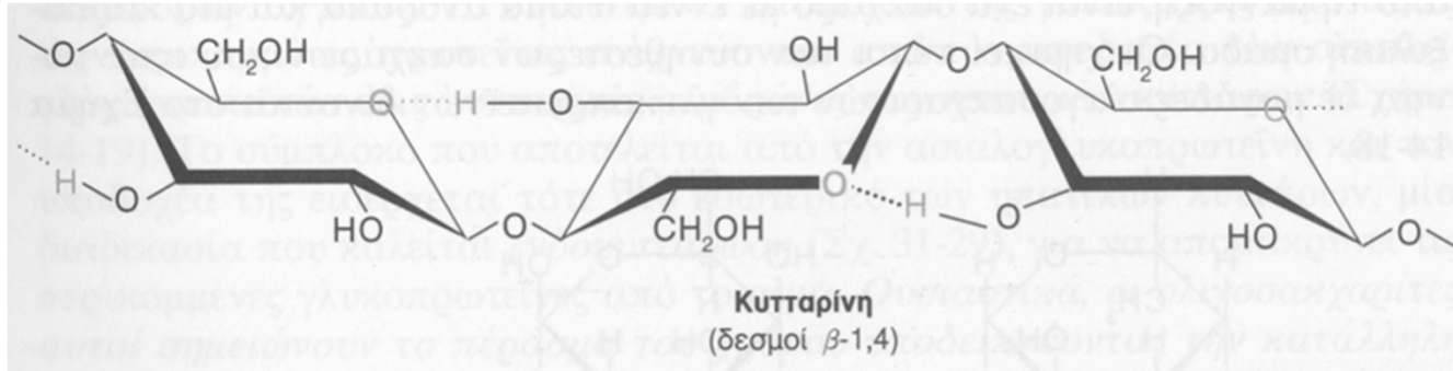
Σχ. 89. Δομή κυτταρίνης.
