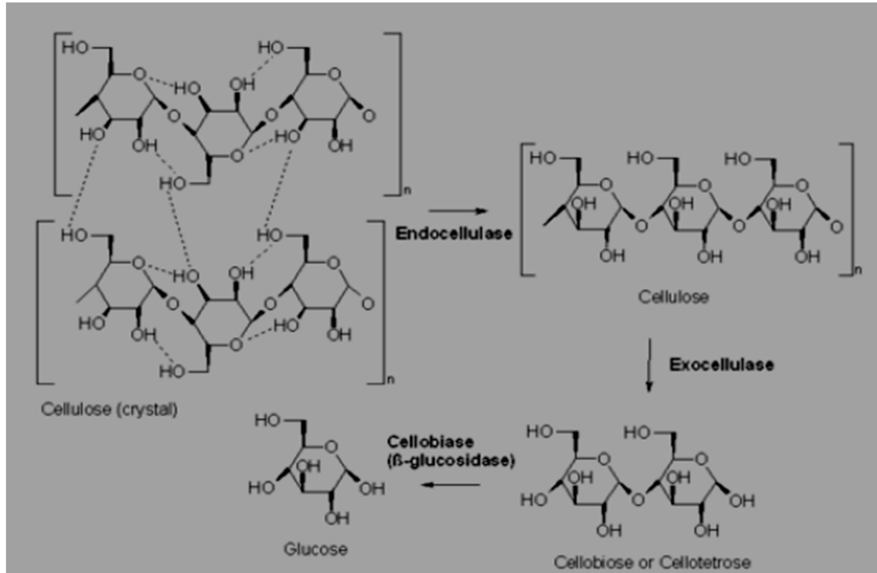
Σχ. 90. Ενζυματική διάσπαση κυτταρίνης.
