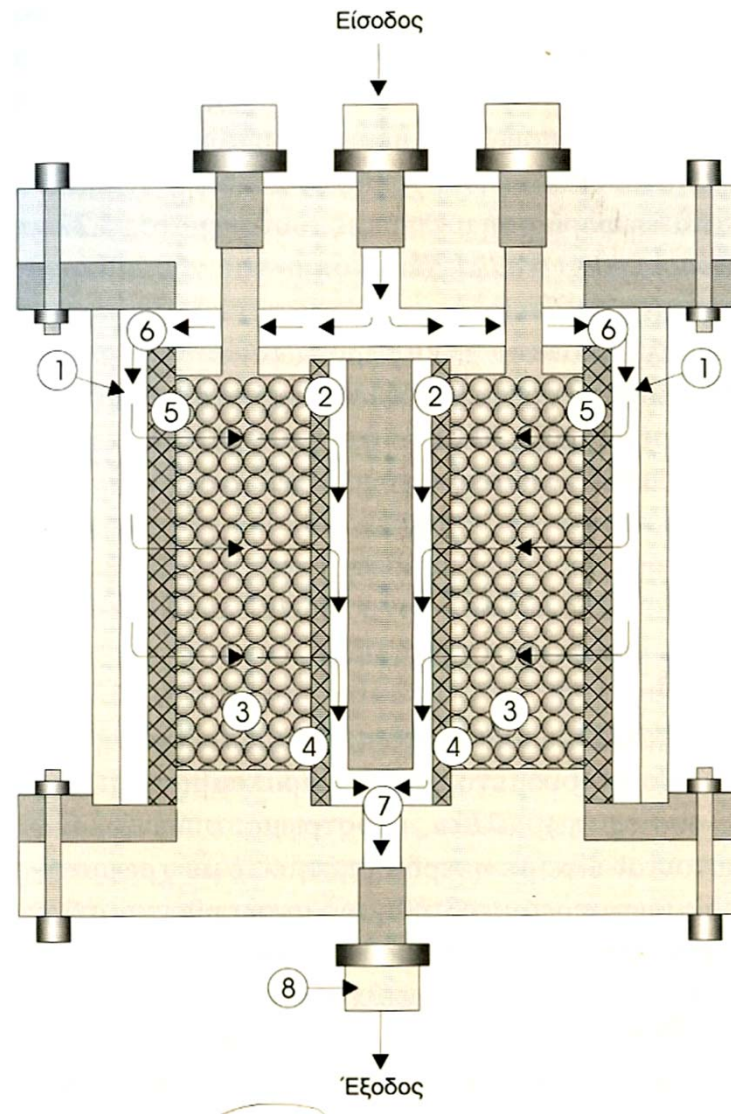
Σχ. 21. Στήλη ακτινικής ροής: (1) διάυλος εισόδου δείγματος, (2) εσωτερικός διάυλος εξόδου εκλούσματος από το χρωματογραφικό υλικό, (3) χρωματογραφικό υλικό, (4) και (5) πορώδεις επιφάνειες (πλέγμα) συγκράτησης χρωματογραφικού υλικού, (6) διανεμητής δείγματος, (7) περιοχή συλλογής εκλούσματος και (8) διάυλος εξόδου από τη στήλη.
