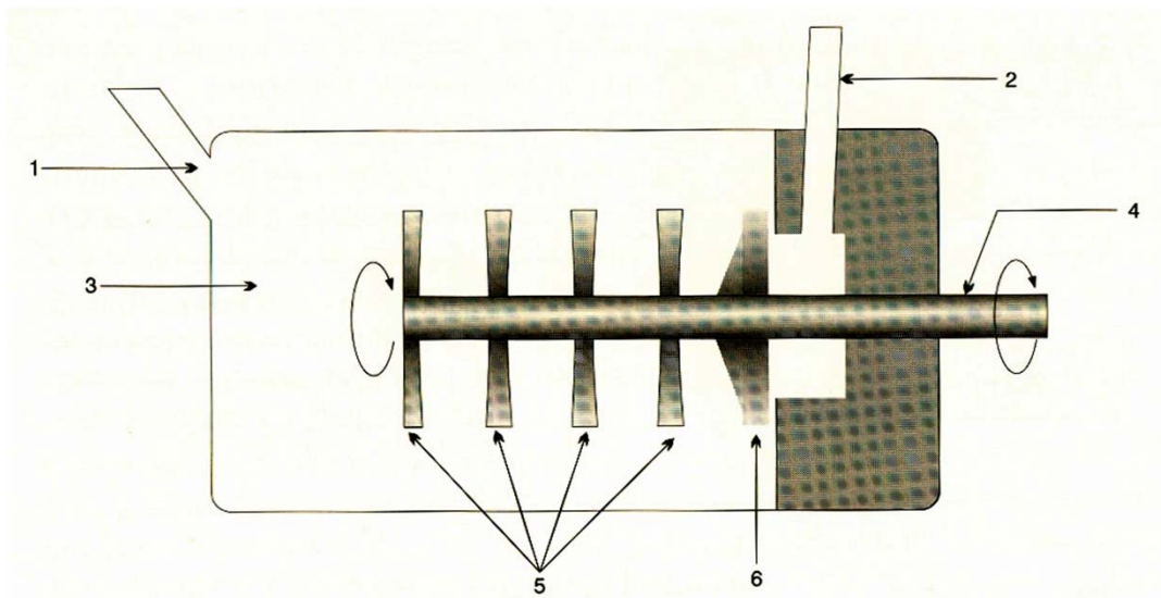
Σχ.6. Μηχανικός θρυμματιστής. (1) Είσοδος, (2) Έξοδος, (3) Δονούμενος κυλινδρικός θάλαμος, (4) Περιστρεφόμενος άξονας, (5) Πτερύγια, (6) Δυναμικός διαχωριστής.
