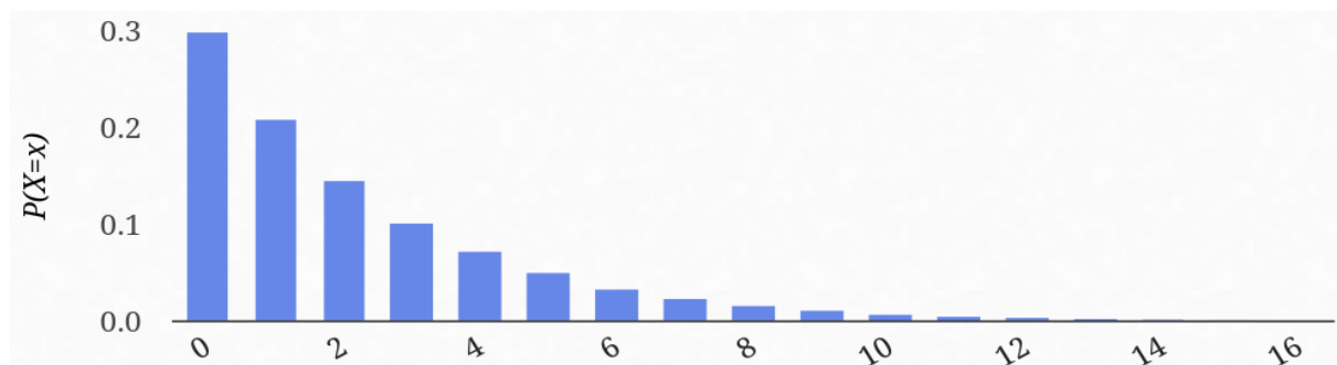
Διάγραμμα 8: Κατανομή πλήθους απογόνων Y \sim \text{Geometric}(0,3)
