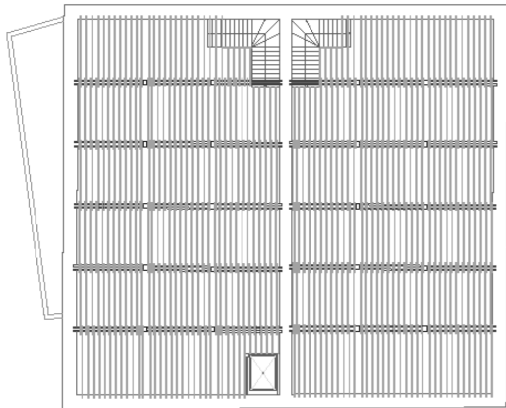
Ανόψη κατασκευαστικής δομής ισογείου
