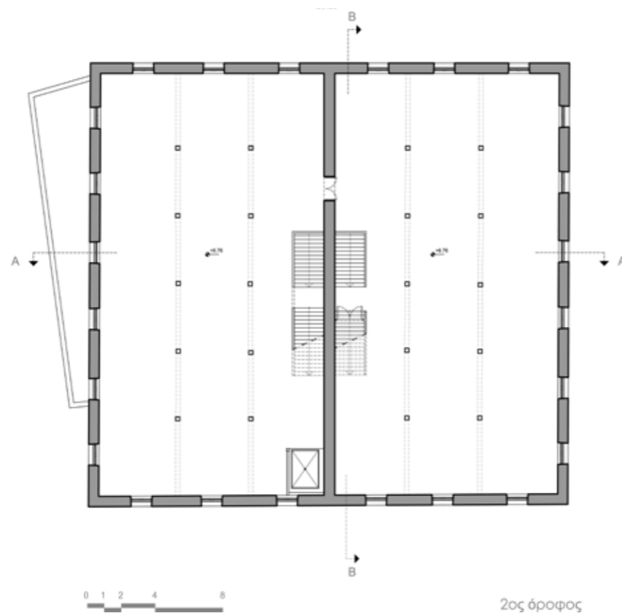
Η καπναποθήκη Τσιμίνο - αποτύπωση Μάρτιος 2014
