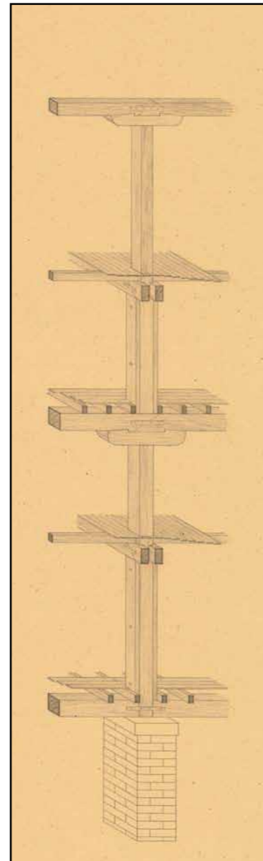
Κατασκευαστικό σύστημα δοκών στύλων καπναποθήκης Πορτοκάλογλου στη Δράμα [διπλωματική εργασία Δ.Π.Θ.]
