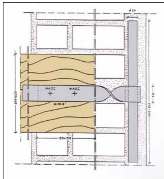
Μεταλλικές λάμες στην τοιχοποιία δένουν την κατασκευή, προσφέροντας αντισεισμική ικανότητα. Στα σχήματα παρουσιάζονται τρόποι σύνδεσης ξύλινης δοκού με την μεταλλική λάμα.
