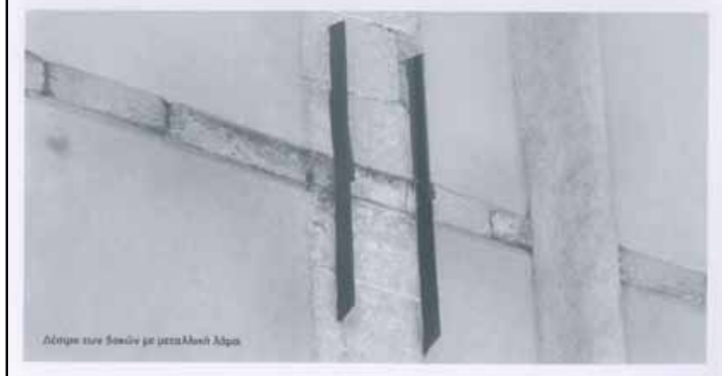
Κατασκευαστικό σχέδιο του αρχιτέκτονα Ιωάννη Τόμπου - αντισεισμική αγκύρωση δοκών και λιθοδομής των καπναποθηκών της Καβάλας. Δέσιμο των δοκών με μεταλλική λάμα.
