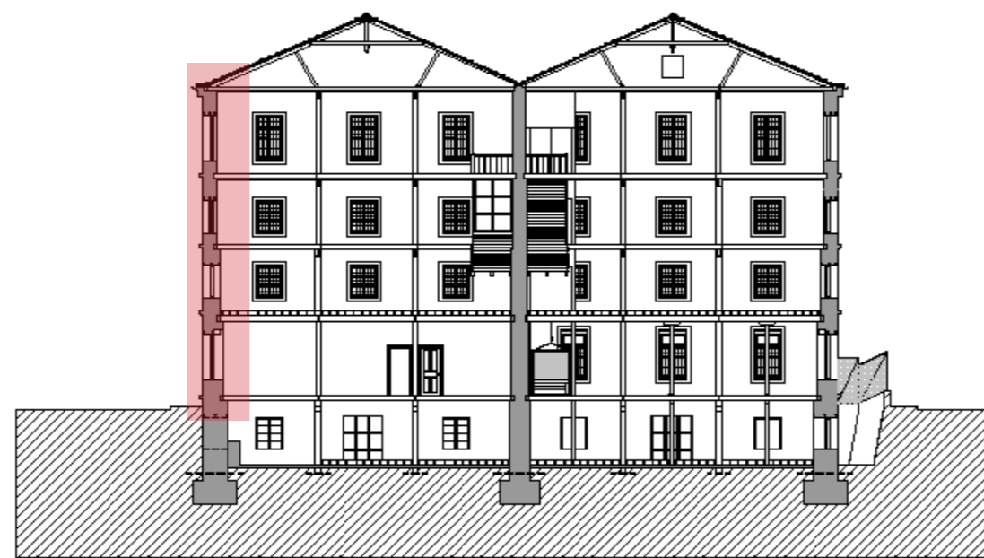
τομή Α-Α'
