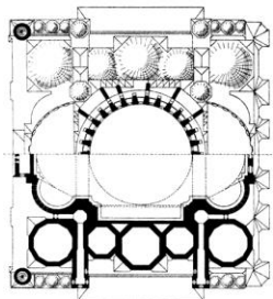
HORIZONTALSCHNITT DURCH DIE TAMBURE DER KLEINEN KUPPELN
