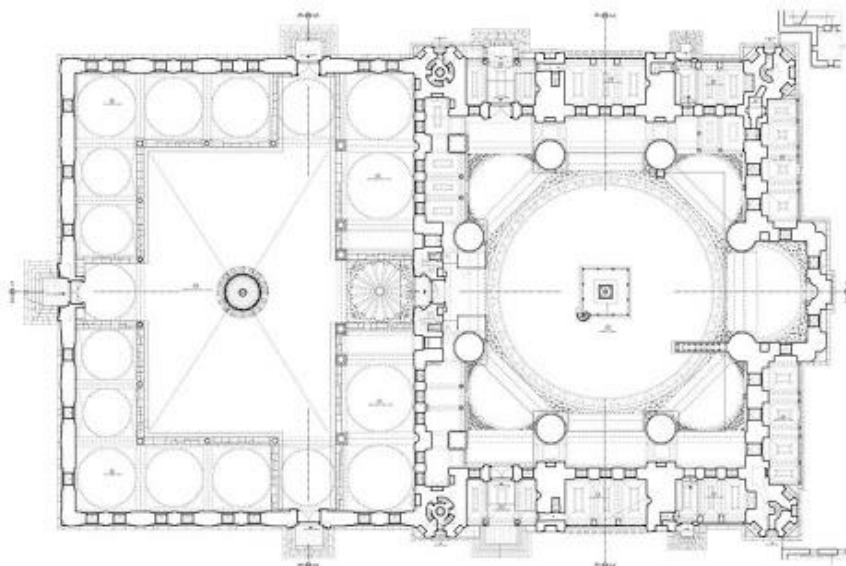
EDİRNE SELİMİYE CAMII • ZEMİN KAT PLANI (1:10 KÖTÜ) • BÖLÜME • ÖLÇEK: 1/50
