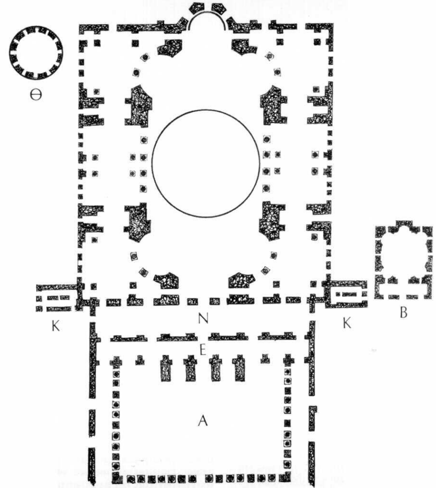
Κάτοψη τής Αγίας Σοφίας
