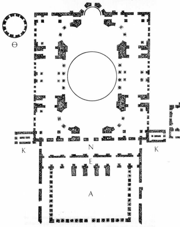
Κάτοψη τής Αγίας Σοφίας
