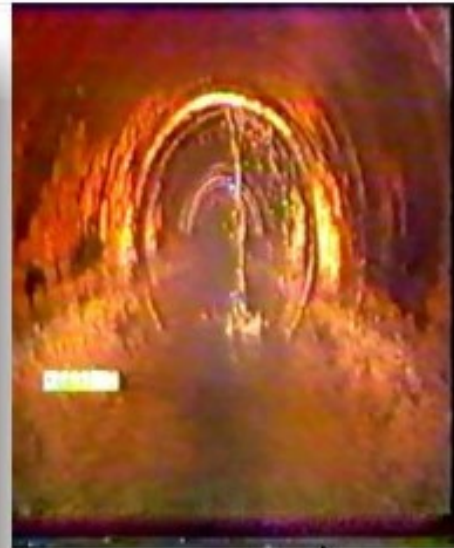
Αρμοί και ρωγμές σε αποχετευτικό αγωγό
