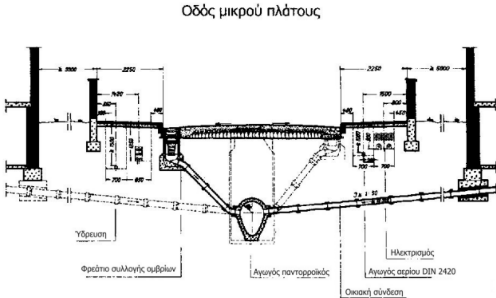
Σχήμα 1.1 : Τυπική διατομή οδού με παντοροϊκό δίκτυο αποχέτευσης
