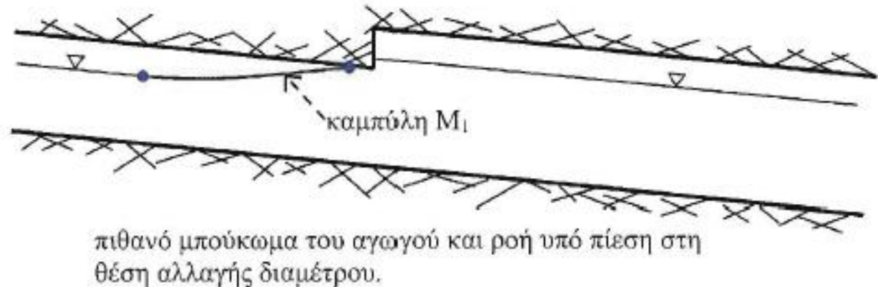
(β) Αλλαγή διαμέτρου αγωγού με ταύτιση πυθμένα
