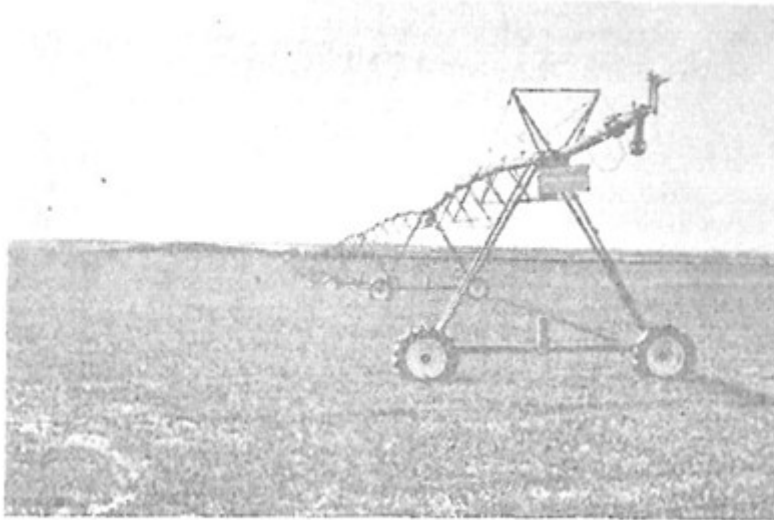
Σχήμα 6: Μετακινούμενες σωληνώσεις
