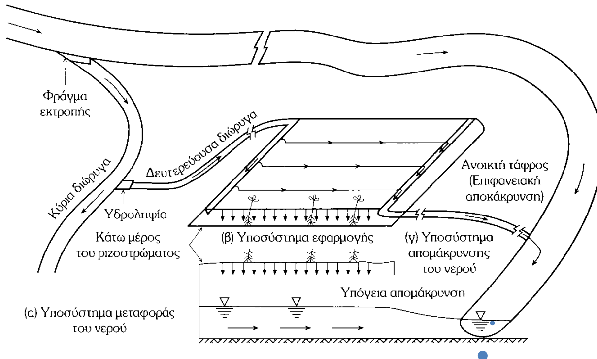
Σχ. 13.2: Διαγραμματική αναπαράσταση του συστήματος ποταμού – αρ- δευόμενης έκτασης – απομάκρυνση νερού.
