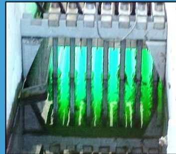
Λυχνίες πολύ χαμηλής πίεσης ατμών Hg. Μαμάσης
