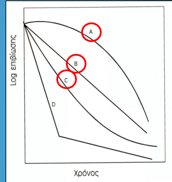
Τύποι καμπυλών επιβίωσης των μικροοργανισμών. Μήτρακας
