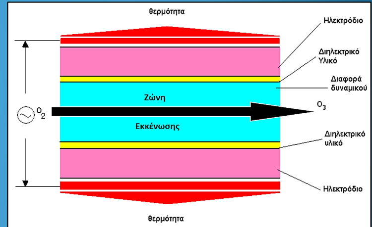
Παραγωγή όζοντος με οζονιστή. Μήτρακας
