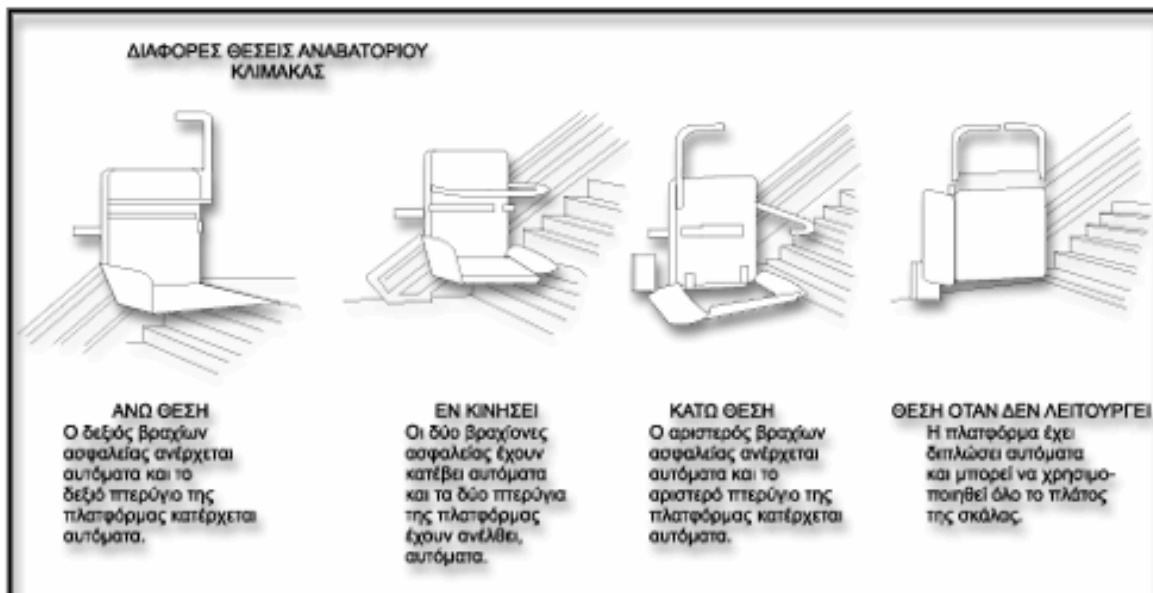
Σχ. 69, Διάφορες θέσεις αναβατορίου κλίμακας
