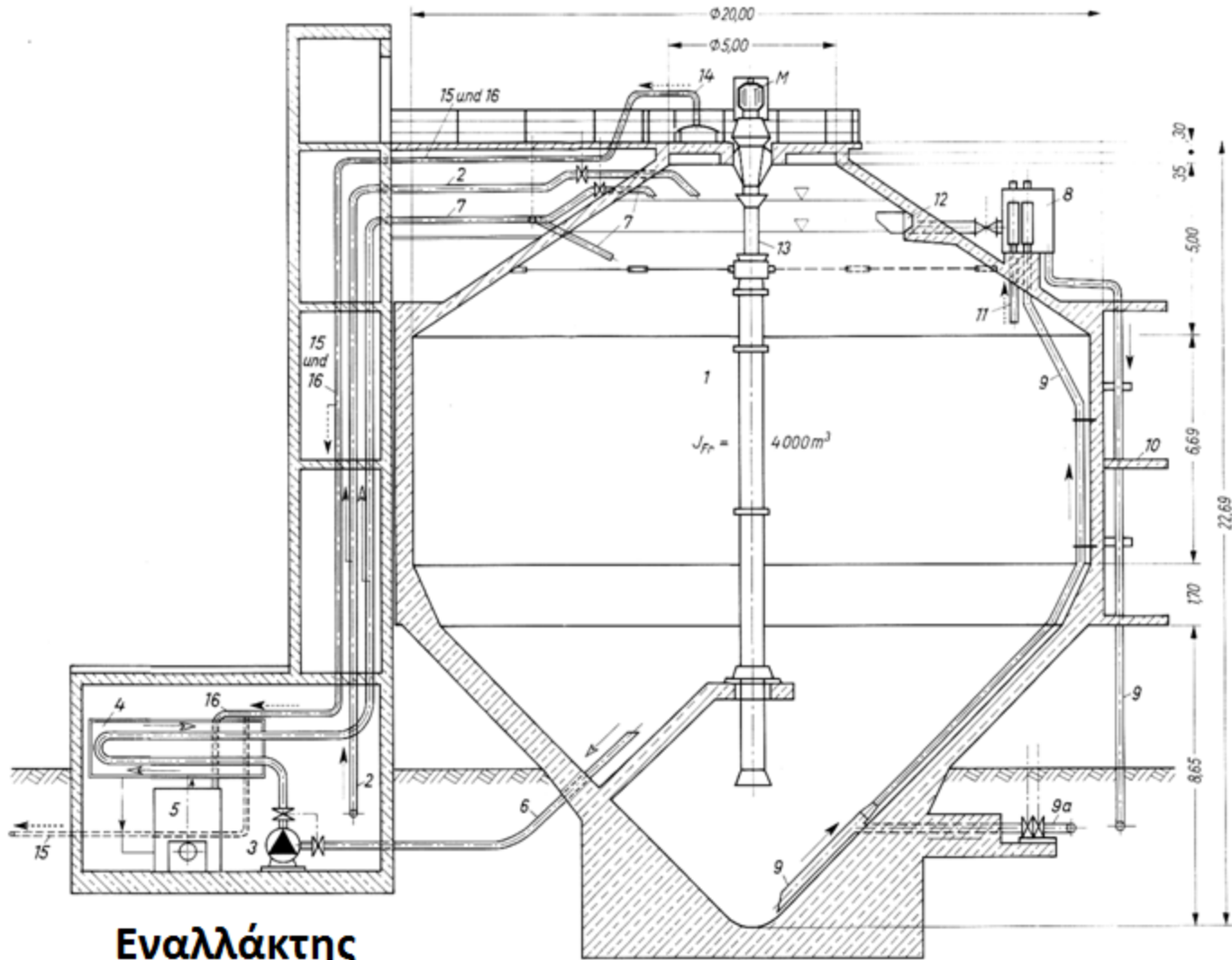
Αναερόβιος χωνευτής
