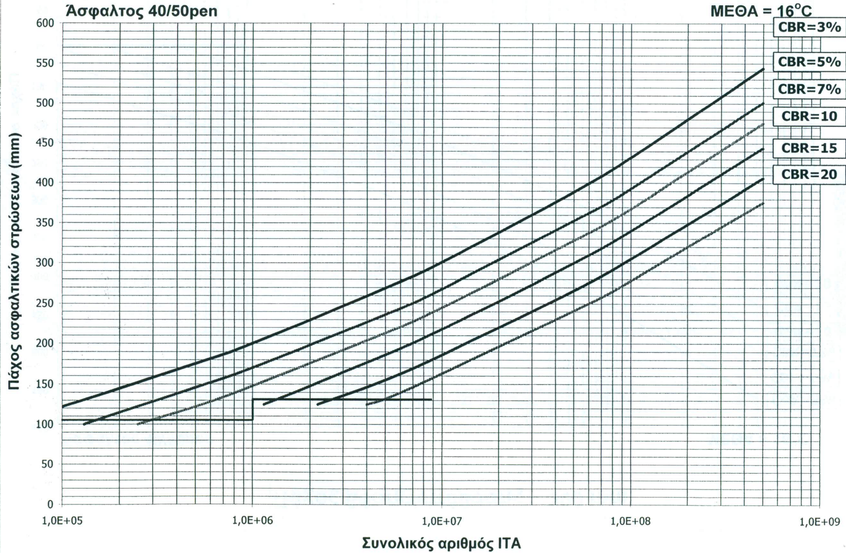
Σχήμα A-10 Νομογράφημα υπολογισμού πάχους ασφαλτικών στρώσεων για πάχος βάσης/υπόβασης 400mm και ΜΕΘΑ 16°C, με άσφαλο 40/50 pen
