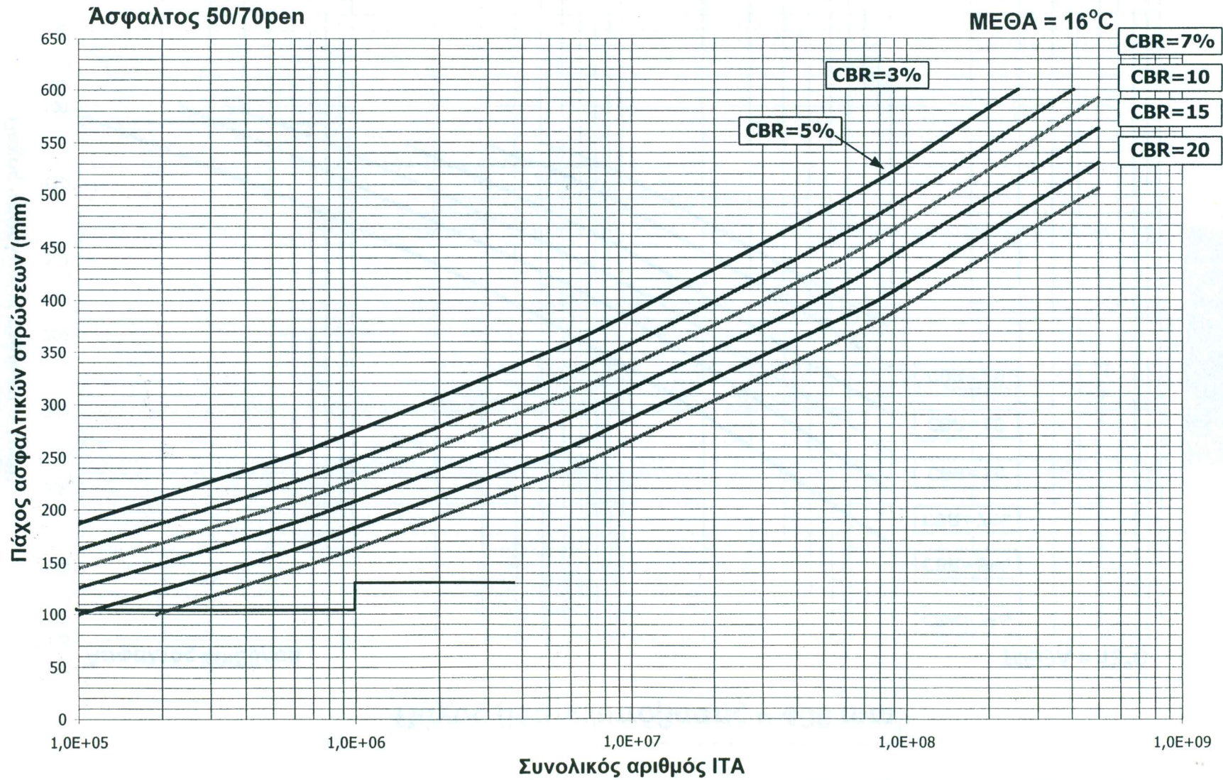
Σχήμα Α-6 Νομογράφημα υπολογισμού πάχους ασφαλτικών στρώσεων για πάχος βάσης/υπόβασης 200mm και ΜΕΘΑ 16°C, με άσφαλτο 50/70pen
