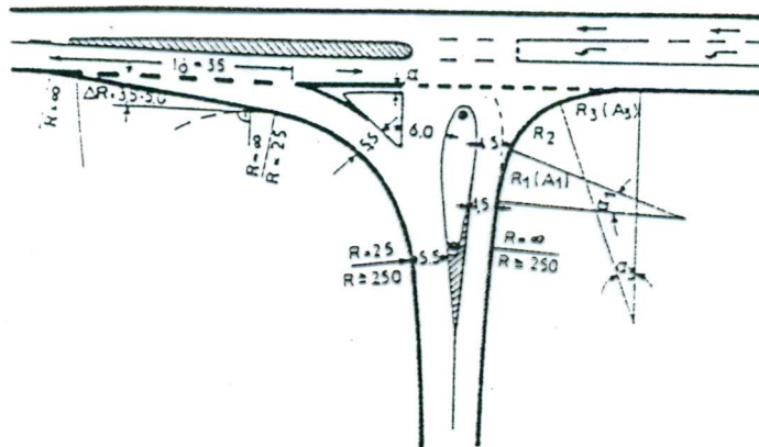
Σχ. 6.13. Γεωμετρική διαμόρφωση κόμβου μορφής ορθής διασταυρώσεως
