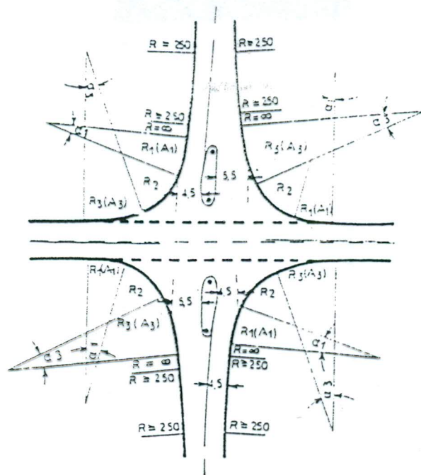
Σχ. 6.12. Γεωμετρική διαμόρφωση κόμβου μορφής ορθής διασταυρώσεως
