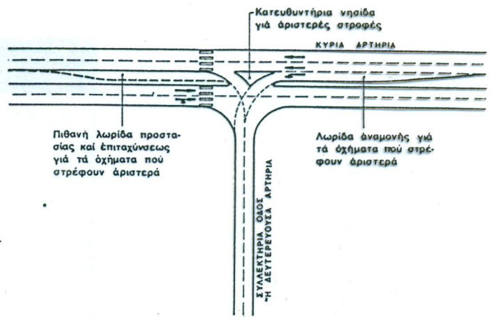
Β. Κόμβος μορφής T με διαχωρισμό κατευθύνσεων και διοχετευτική διαρρύθμιση στη συνεχιζόμενη οδό
