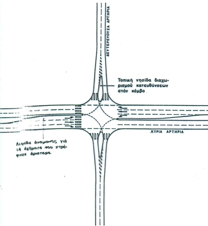
Γ. Κόμβος 4 σκελών με διαχωρισμό των κατευθύνσεων στη μία οδό
