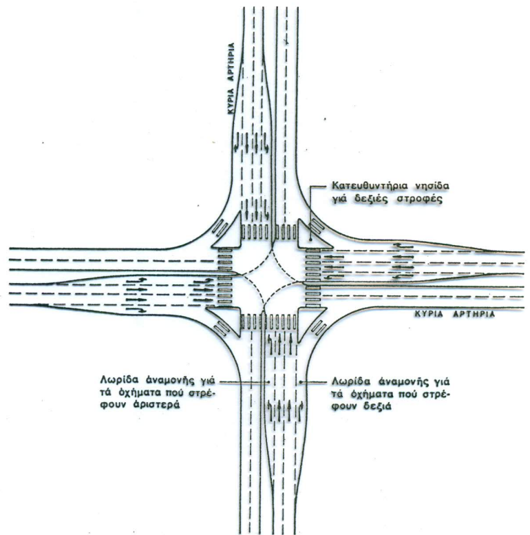
Δ. Κόμβος 4 σκελών με πλήρη διαχωρισμό κατευθύνσεων και έκτεταμένη διοχετευτική διαρρύθμιση
