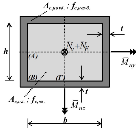
Σχ. Σ8.Α: Μανδύας υποστυλώματος.
