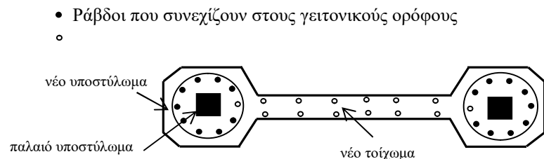
Σχ. Σ8.6: Ενδεικτική εμφάνιση με πάχος ίσο ή μικρότερο του πλάτους της δοκού
