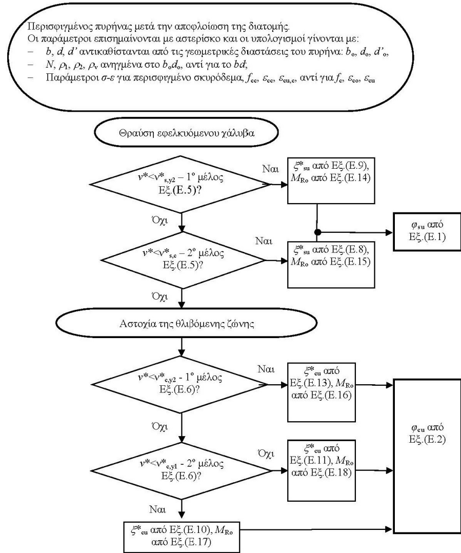
Διάγραμμα ροής 2: Βήματα για τον υπολογισμό της καμπυλότητας αστοχίας περισφιγμένου πυρήνα μετά την αποφλοιώσή της διατομής.
