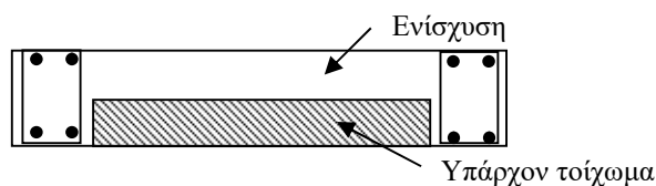
Σχ. Σ8.4: Ενδεικτική διάταξη μονόπλευρης ενίσχυσης τοιχώματος
