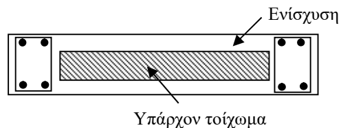
Σχ. Σ8.5: Ενδεικτική διάταξη ολόπλευρου κλειστού μανδύα ενίσχυσης τοιχώματος
