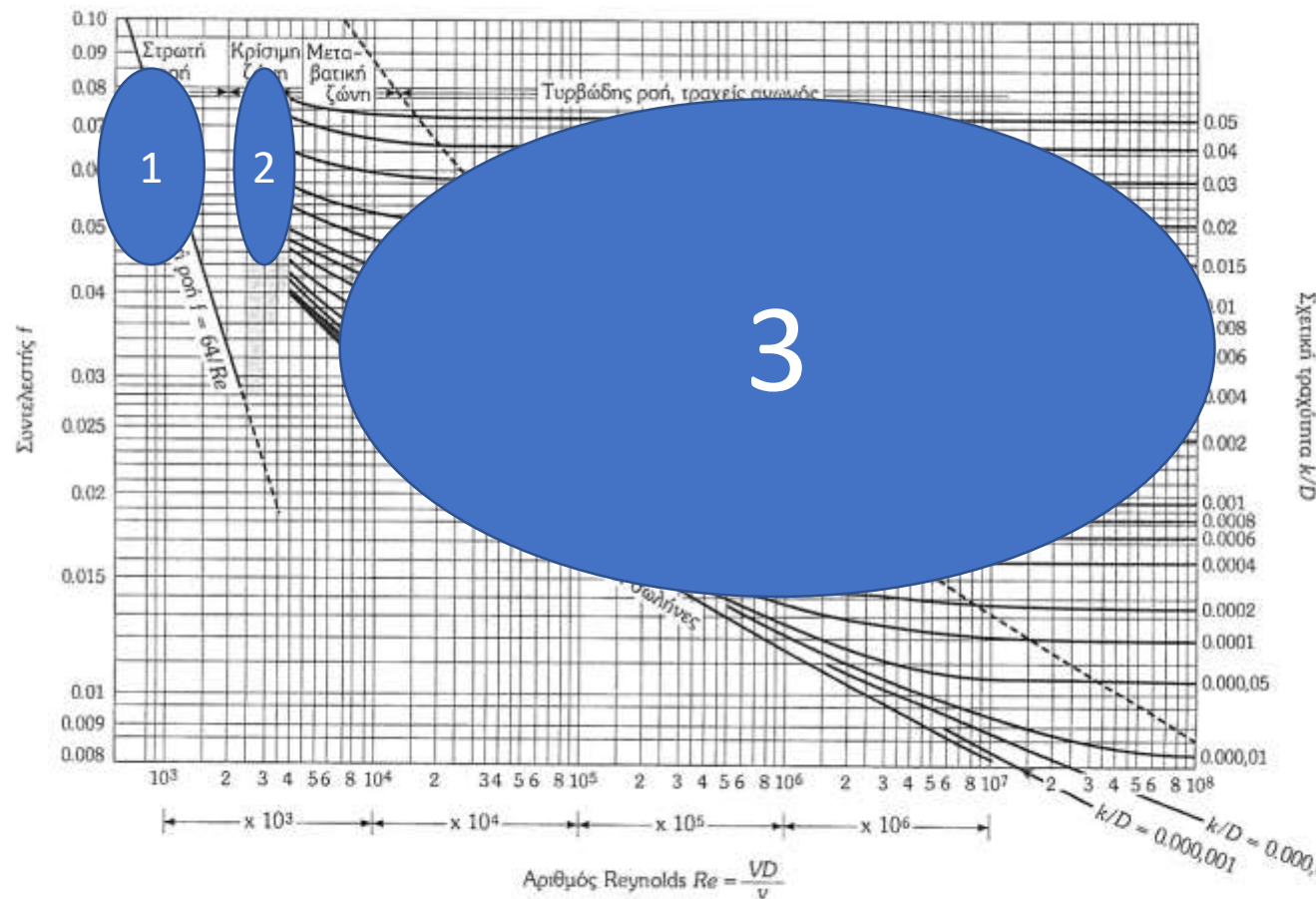
Σχ. 2.2: Διάγραμμα Moody.
