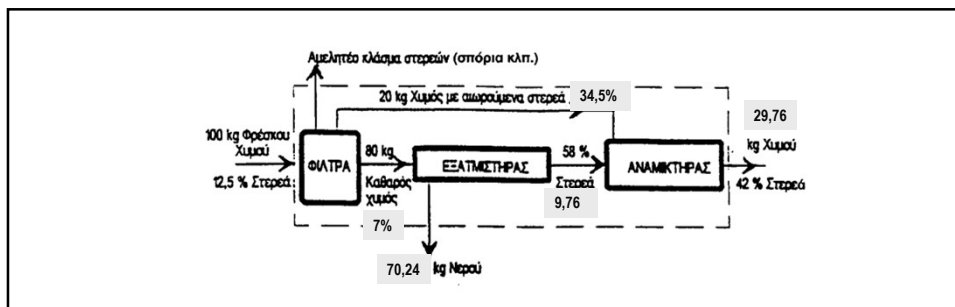
Σχ. 2.5. Γραμμή παραγωγής συμπυκνωμένου πορτοκαλοχυμού
