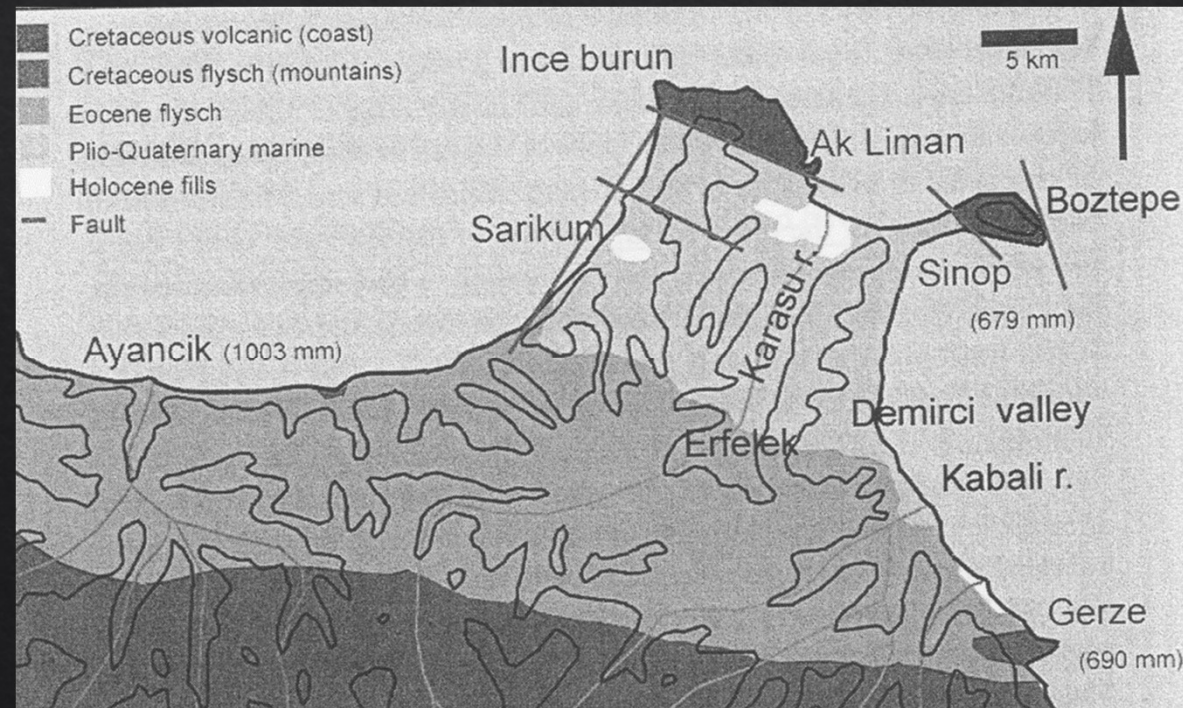
Γεωλογικές ζώνες της χερσονήσου της Σινώπης
