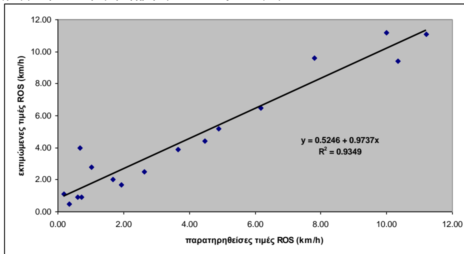
Σχήμα 2: Συσχέτιση εκτιμώμενων και πραγματικών τιμών ROS επιφάνειας Figure 2: Correlation of ROS_{estimated(surface)} and ROS_{observed} values
