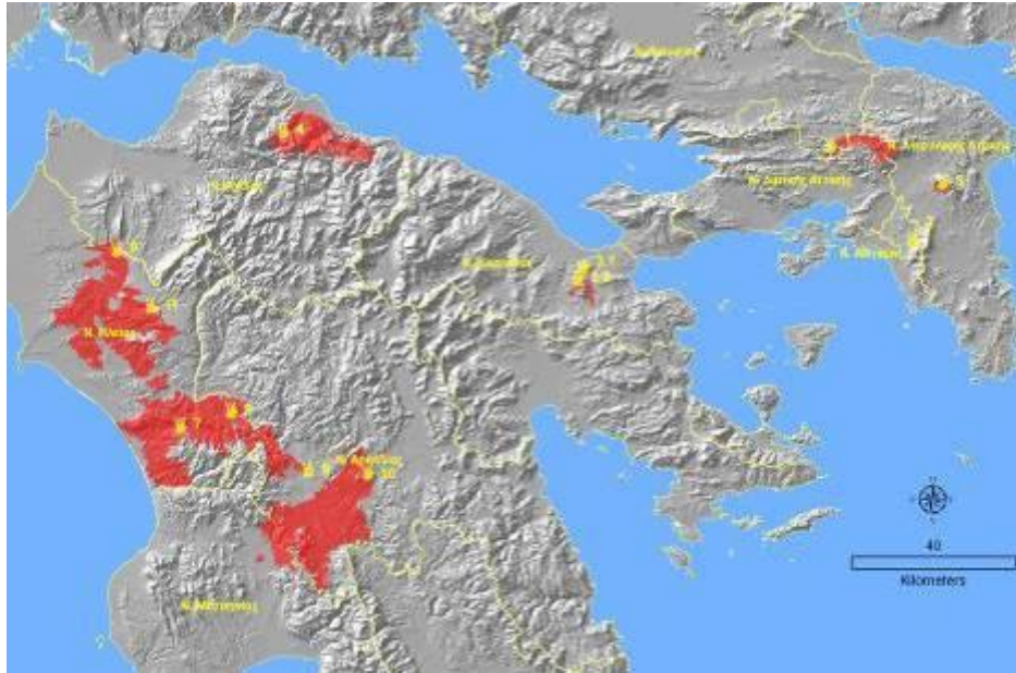
Σχήμα 1: Καμμένες εκτάσεις των δώδεκα τεκμηριωμένων δασικών πυρκαγιών Figure 1: Burned areas of twelve documented forest fires
