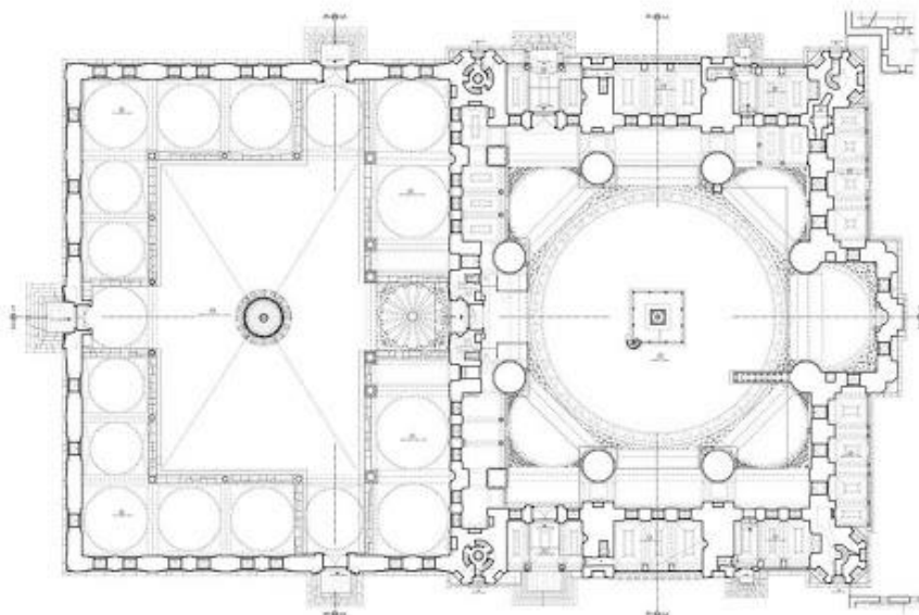
EDİRNE SELİMİYE CAMII • ZEMİN KAT PLANI (LİH KÖTÜ) • BÖLÜME • ÖLÇEK: 1/50
