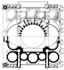
HORIZONTALSCHNITT DURCH DEN TAMBUR DER HAUPTKUPPEL
