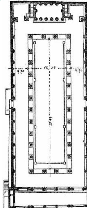
Κάτοψη Βασιλικής Πομπηίας
