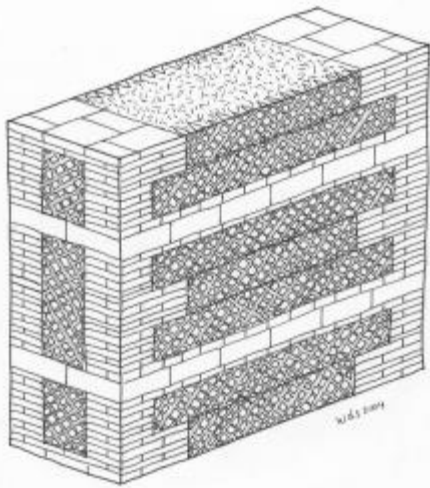
Opus mixtum
