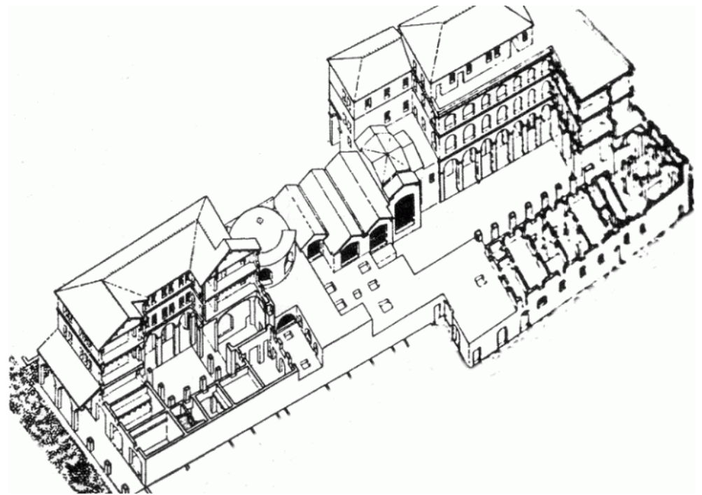
Reconstruction drawing by Italo Gismondi. From left to right: Caseggiato del Serapide (House of Serapides), Terme dei Sette Sapienti (Baths of the Seven Sages), Cas. degli Aurighi (House of the Charioteers)
