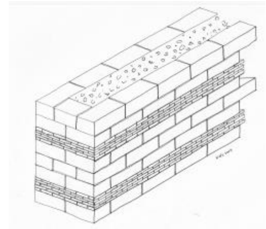
Opus vittatum
