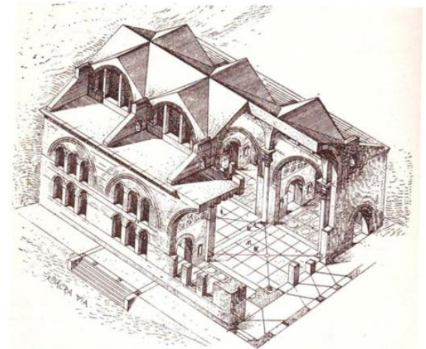
5. 'Η βασιλική του Μαξεντίου και του Κωνσταντίνου στην Ρώμη, σε αποκατάσταση (Durm).
