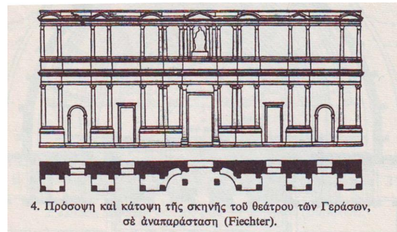
5. Πρόσοψη, κάτοψη και τομή της σκηνής του θεάτρου της Σαγαλασσού, σε αναπαράσταση (Croma).
