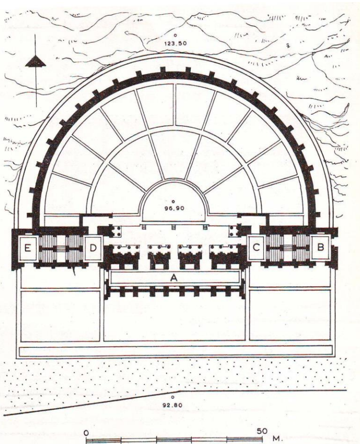
3. Κάτοψη του Ὁδείου Ἡρώδου τοῦ Ἀττικοῦ, σὲ ἀναπαράσταση (Τραυλός).
