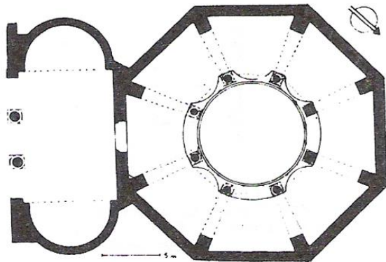
Roma. Battistero di S. Giovanni al Laterano, c. 315, c. 432–40, pianta e ricostruzione assometrica nel 320
