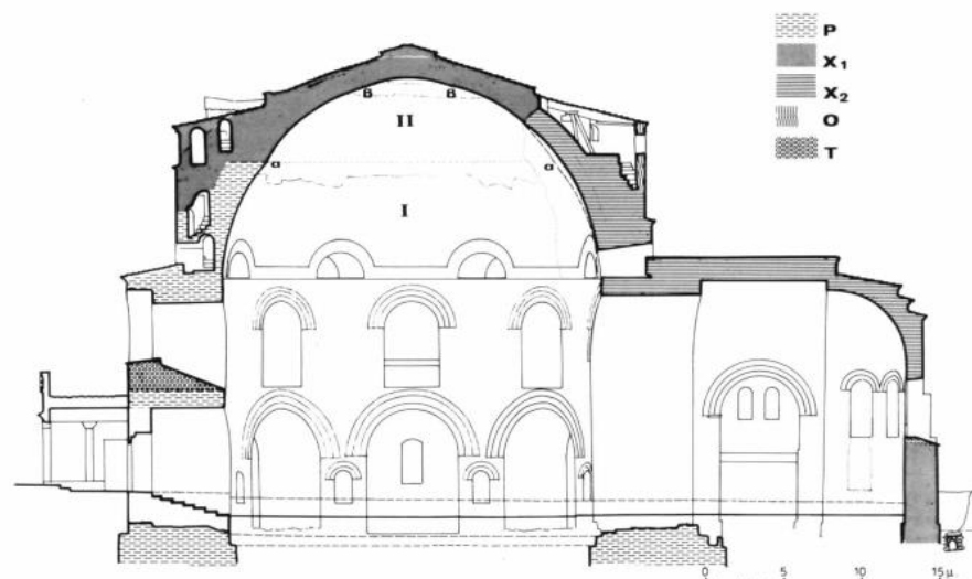
Εικ. 11. Τομή κατά μήκος, διάκριση φάσεων: P = Ρωμαϊκή φάση. X1 = Παλαιохριστιανικές φάσεις. X2 = Φάση 7ου αι.
