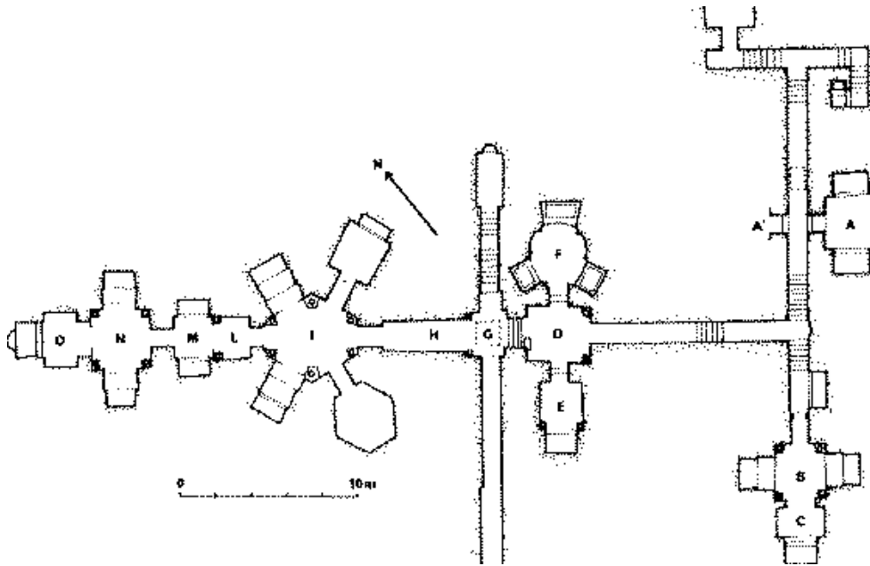
Ρώμη. Κάτοψη της κατακόμβης της Via Latina
