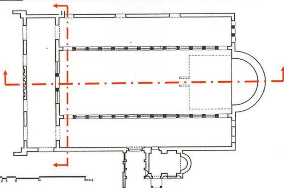
Τρίκλιτη βασιλική Κάτοψη, Τομή κατά μήκος & πλάτος Η Αχειροποίητος Θεσσαλονίκης σε αναπαράσταση (Α. Ορλάνδος)
