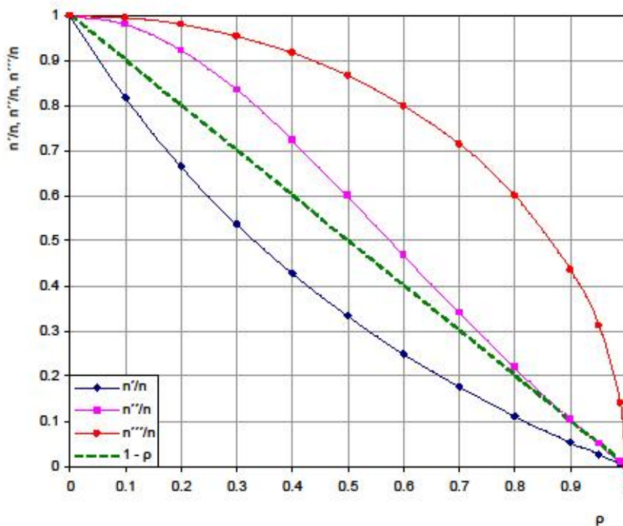
Σχήμα 4.1 Ισοδύναμο μήκος n' , n'' , n''' της πληροφορίας που προσθέτει η δεύτερη μεταβλητή από δείγμα μήκους n στο αρχικό δείγμα επίσης μήκους n , ως συνάρτηση του συντελεστή συσχέτισης των δύο μεταβλητών \rho (εξισώσεις (4.30), (4.36), (4.41), αντίστοιχα).
